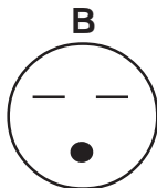
15 AMP 230 VOLT NEMA 6-15P
