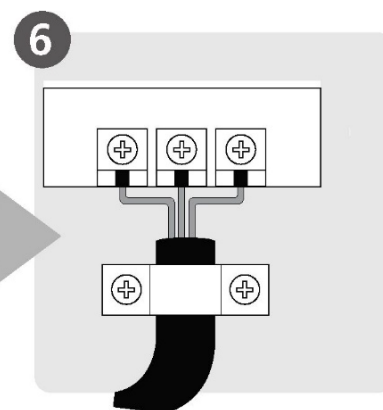
Faites l'installation électrique (non applicable pour certaines régions d'Amérique du Nord)
