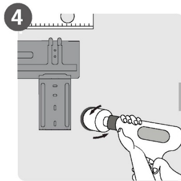
Percez le trou dans le mur
