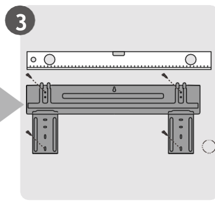
Fijar la placa de montaje
