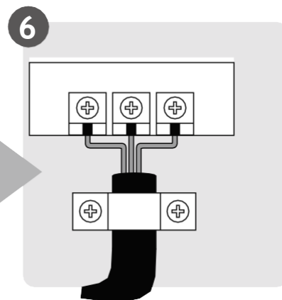
Conectar los cables (no se aplica a algunos lugares de América del Norte)
