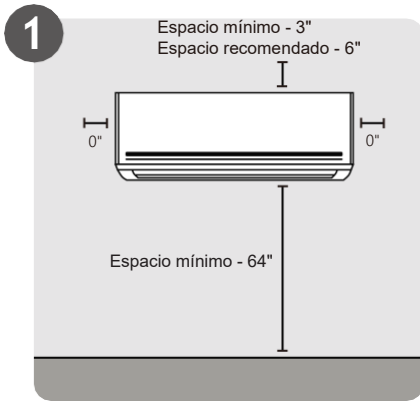
Elegir el lugar de la instalación
