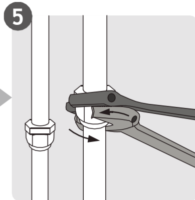
Conectar la tubería
