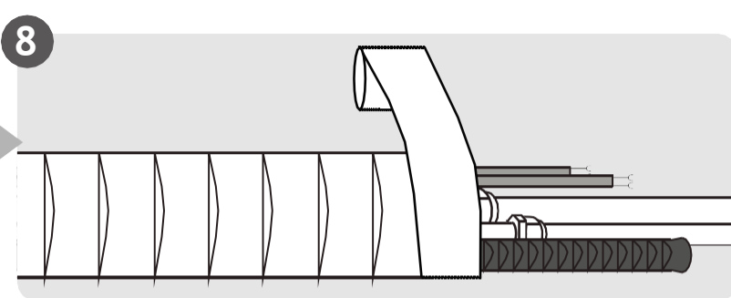
Envolver la tubería y los cables (no se aplica a algunos lugares de América del Norte)
