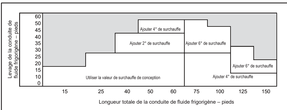
60K AC avec TXV
