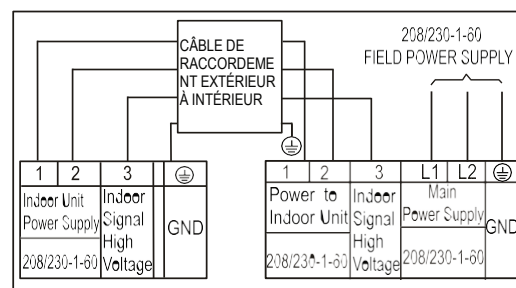
Schéma de connexion (208/ 230V)
