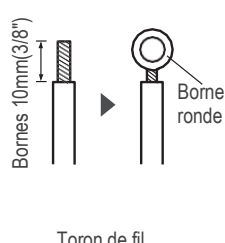
Toron de fil
