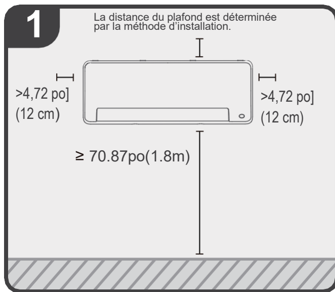
Choisir le lieu de l'installation
