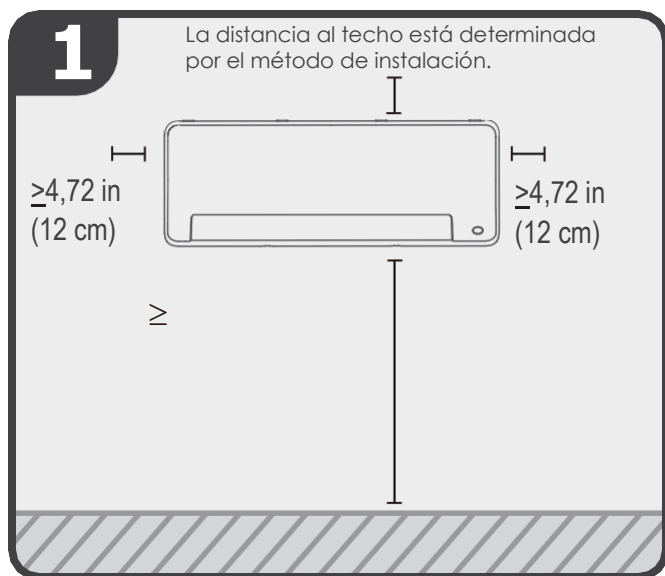
Elegir el lugar de la instalación
